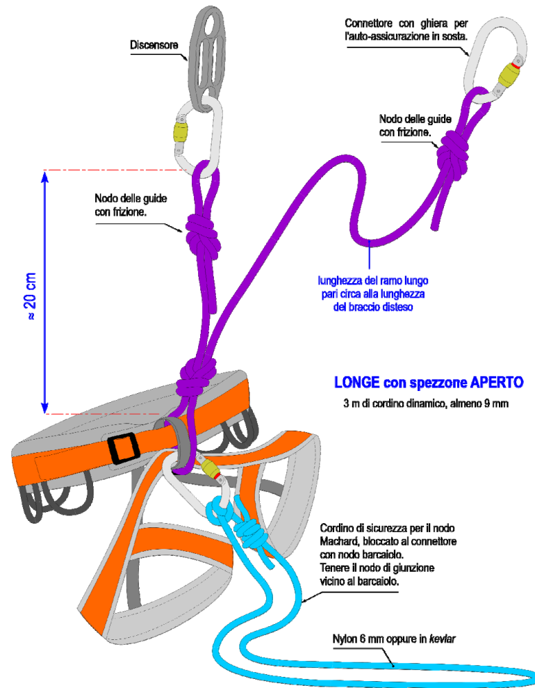
Figura 2(c) – Realizzazione della "longe" per l'auto-assicurazione e la calata con spezzone dinamico aperto.
